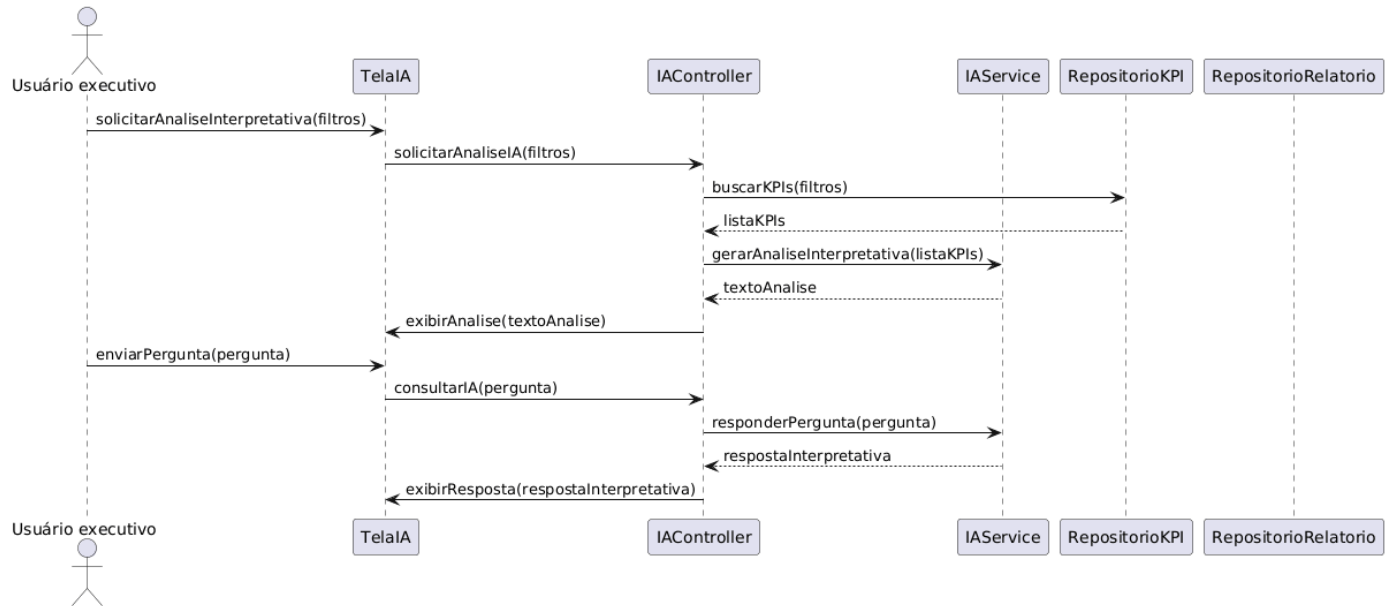
Figura 23. Diagrama de sequência de projeto – UC12/UC13
